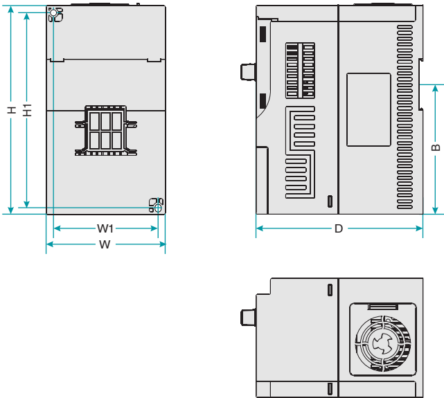
图2-4 变频器外形尺寸及安装尺寸
