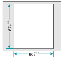
图2-7 键盘不带底座安装开孔尺寸图
