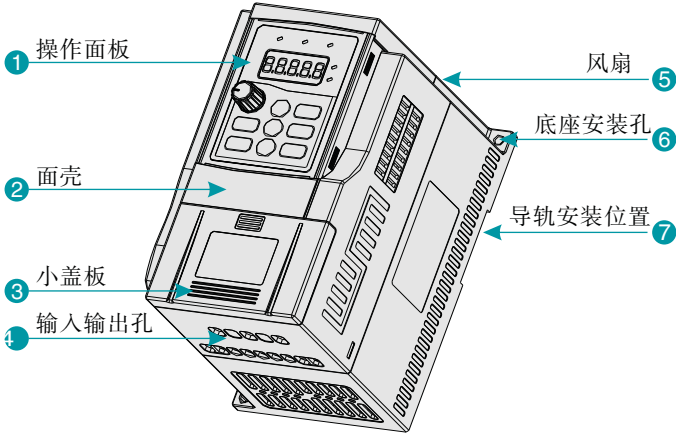
图 2-3 变频器外形图
