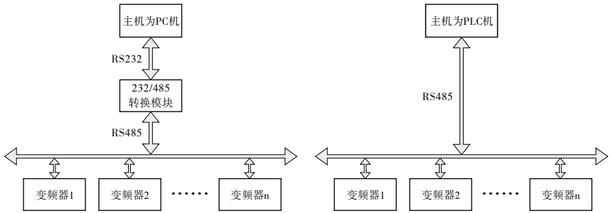
图 7-2 单主机多从机组网方式图
