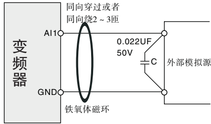
图 3-8 模拟量输入端子处理接线图
