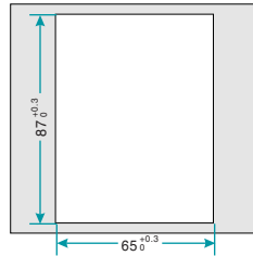
图2-6 键盘带底座安装开孔尺寸图
