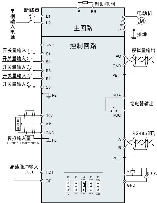
图3-4 基本接线示意图 (2)
