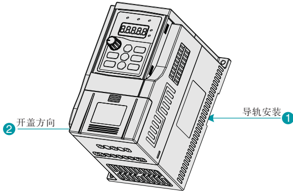
图3-2 塑胶外壳下盖板拆卸图
