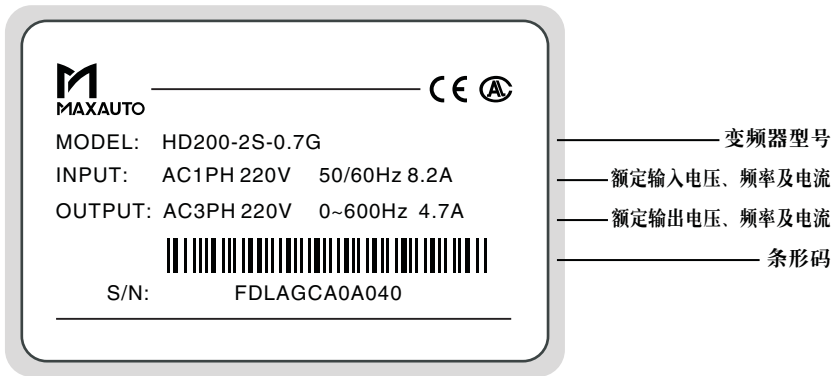
图 2-2 产品铭牌
