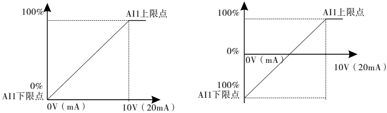
A11输入模拟量对应曲线图
