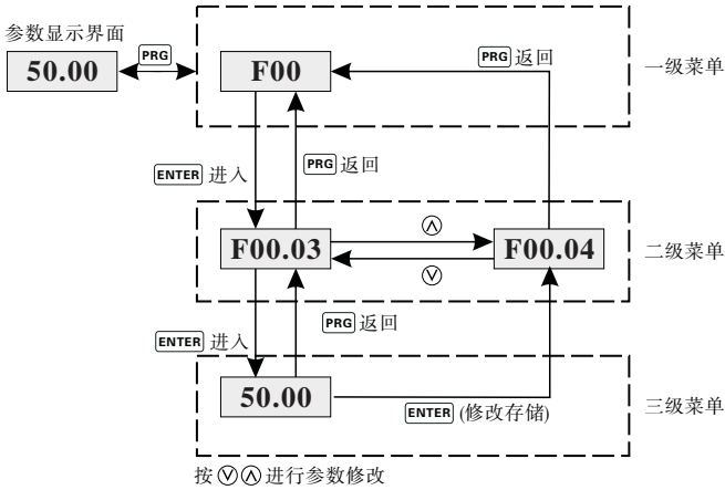
图 4-2 三级菜单操作流程图
