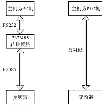
图 7-1 单主机单从机组网方式图
