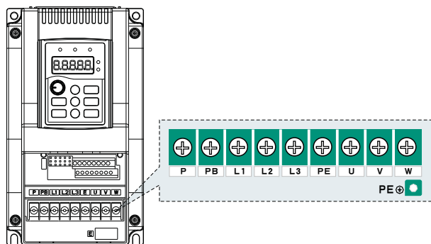
图 3-5 HD200主回路端子示意图
