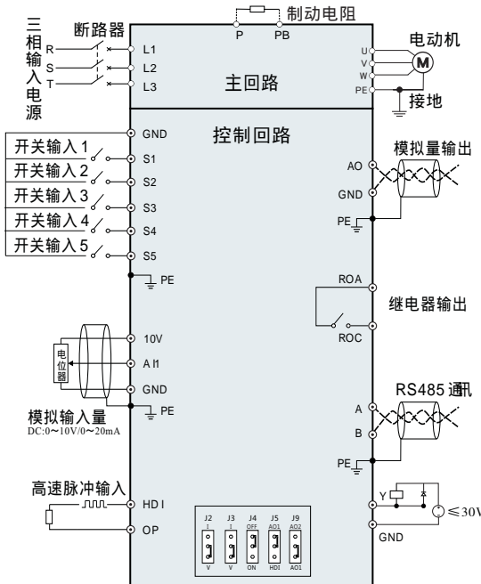
图3-3 基本接线示意图 (1)
