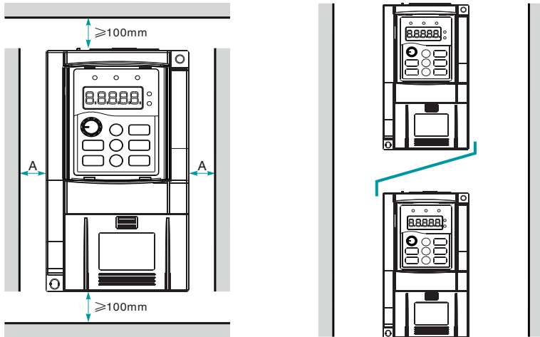
单体安装图
