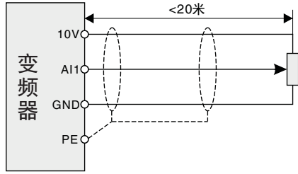
图 3-7 模拟量输入端子接线示意图
