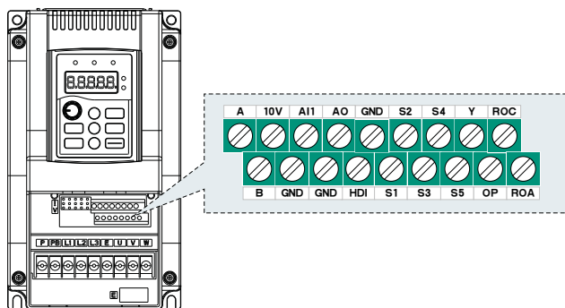
图 3-6 HD200控制回路端子示意图
